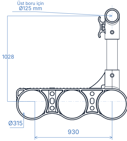
01 ÖNDEN GÖRÜNÜŞ
