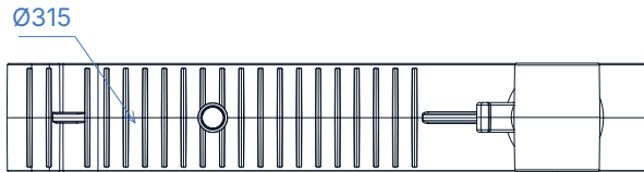
04 ÜSTTEN GÖRÜNÜŞ
