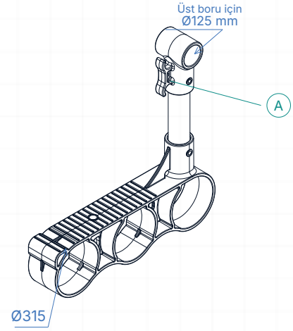
03 İZOMETRİK GÖRÜNÜŞ
