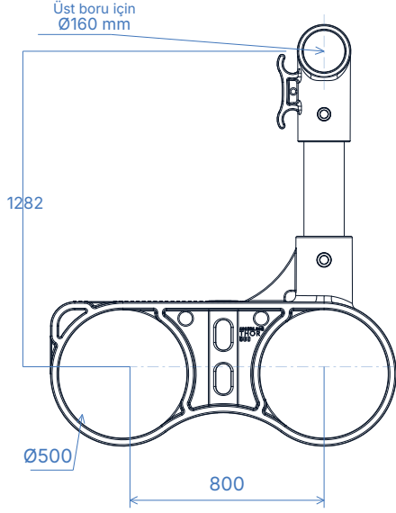
01 ÖNDEN GÖRÜNÜŞ
