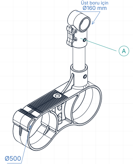
03 İZOMETRİK GÖRÜNÜŞ
