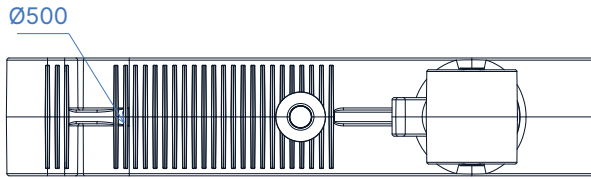
04 ÜSTTEN GÖRÜNÜŞ
