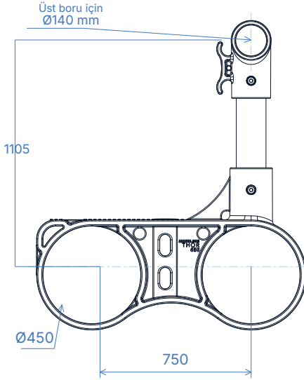
01 ÖNDEN GÖRÜNÜŞ
