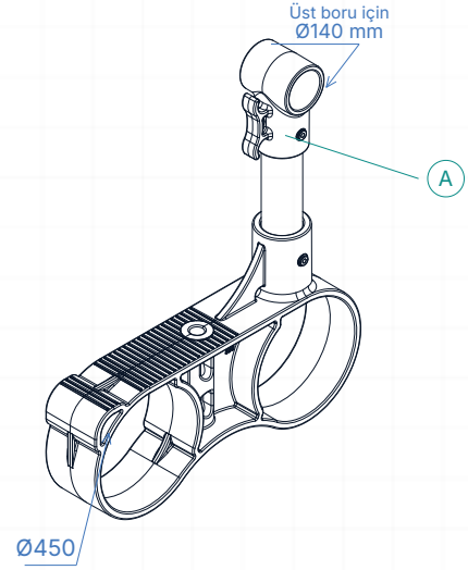
03 İZOMETRİK GÖRÜNÜŞ
