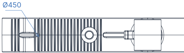
04 ÜSTTEN GÖRÜNÜŞ
