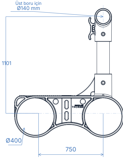
01 ÖNDEN GÖRÜNÜŞ
