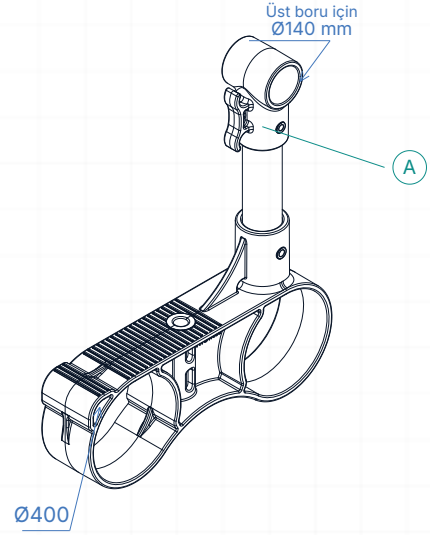
03 İZOMETRİK GÖRÜNÜŞ
