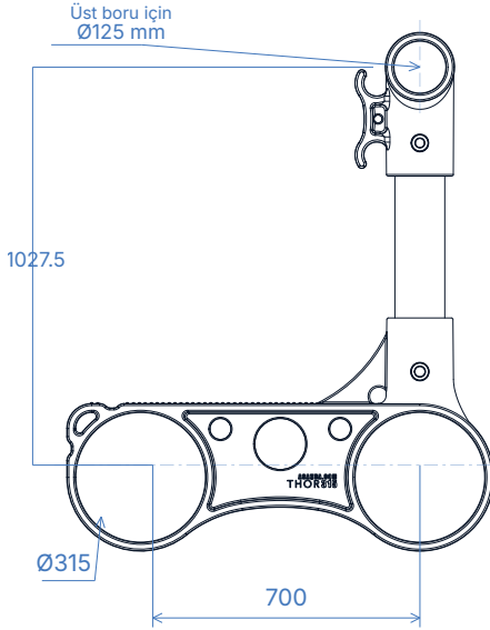
01 ÖNDEN GÖRÜNÜŞ
