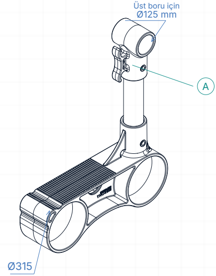
03 İZOMETRİK GÖRÜNÜŞ
