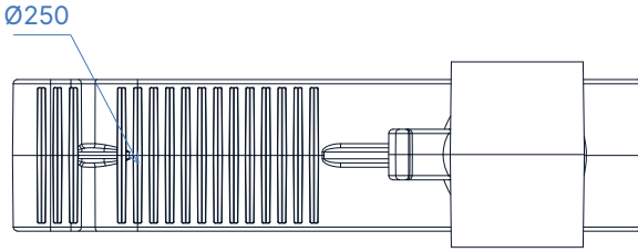
04 ÜSTTEN GÖRÜNÜŞ
