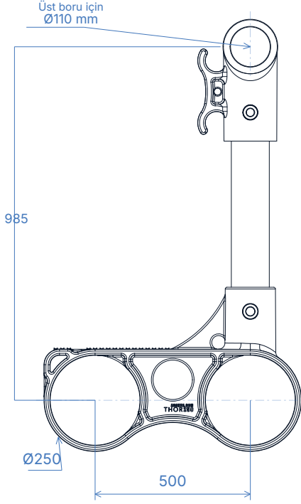
01 ÖNDEN GÖRÜNÜŞ
