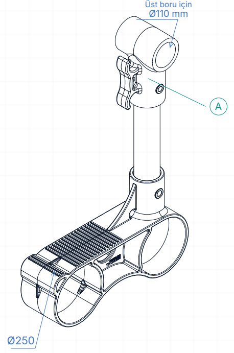
03 İZOMETRİK GÖRÜNÜŞ
